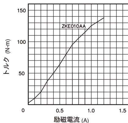
【許容スリップトルク特性図】
