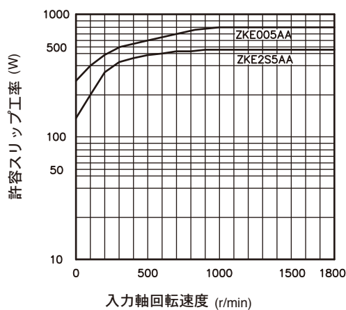
【許容スリップエ率特性図】
