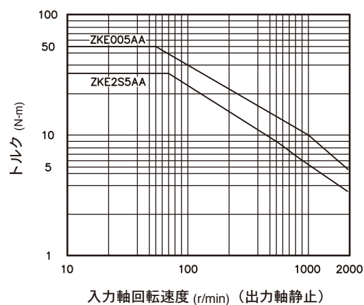
【許容スリップトルク特性図】
